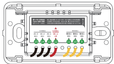
開關背面
